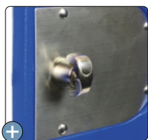
Morillon débrayable assurant une meilleure résistance à l'effraction par rotation
