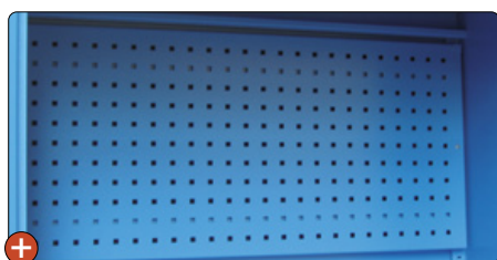
Panneau perforé pour support-outils Perforations carrées 10 x 10 au pas de 38 mm
